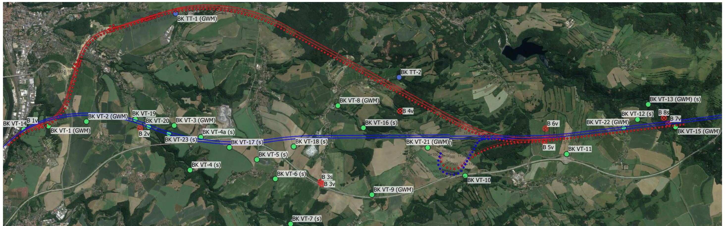
Lageplan mit Voll- und Teiltunnelvariante sowie Aufschlusspunkten 1. und 2. Bohrkampagne
